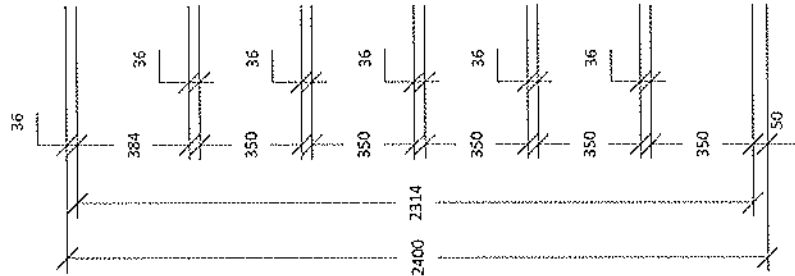
POHLED A-A'
