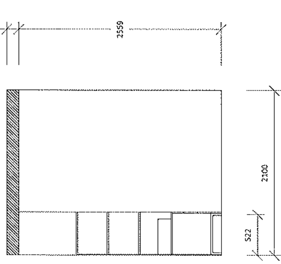
POHLED B
