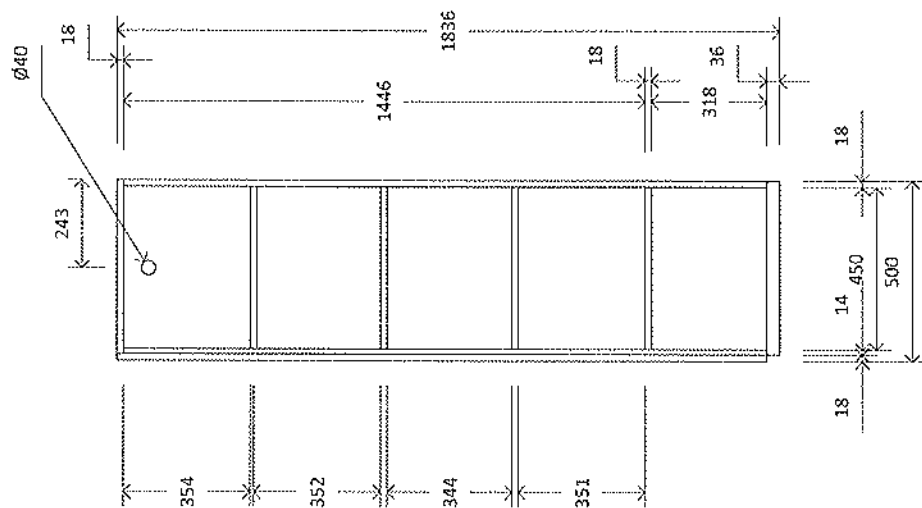
POHLED B-B'
