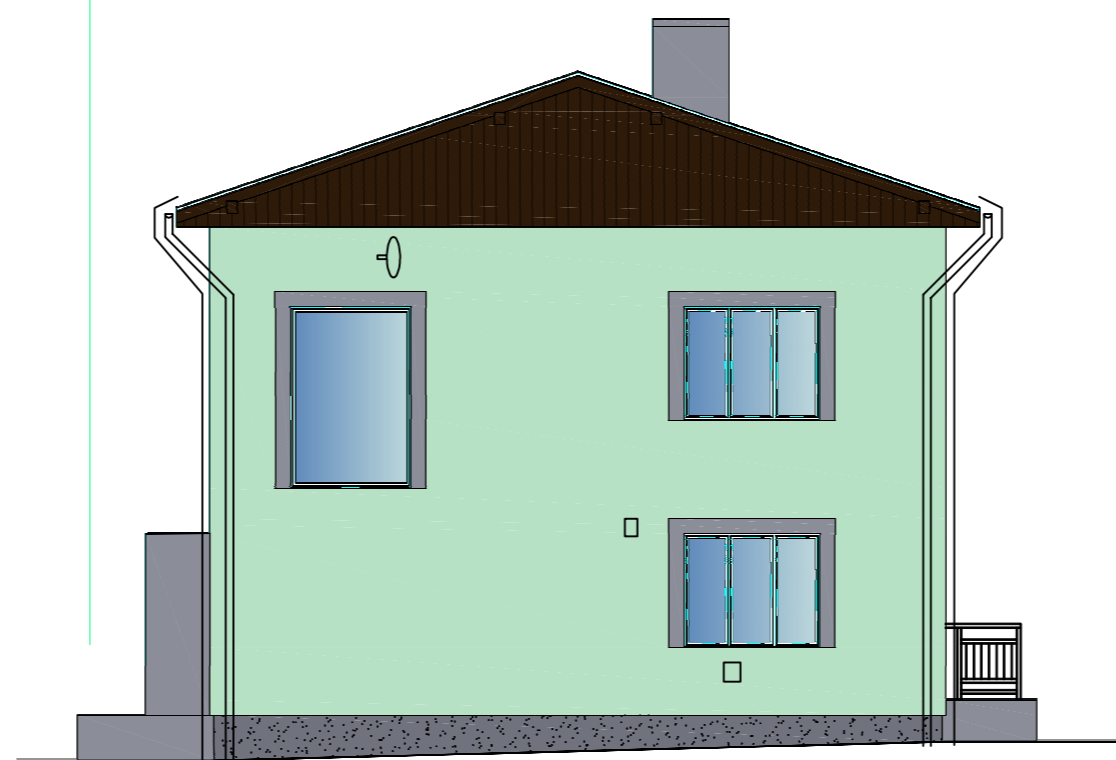
POHLED JIHO-ZÁPADNÍ - BAREVNÉ ŘEŠENÍ
