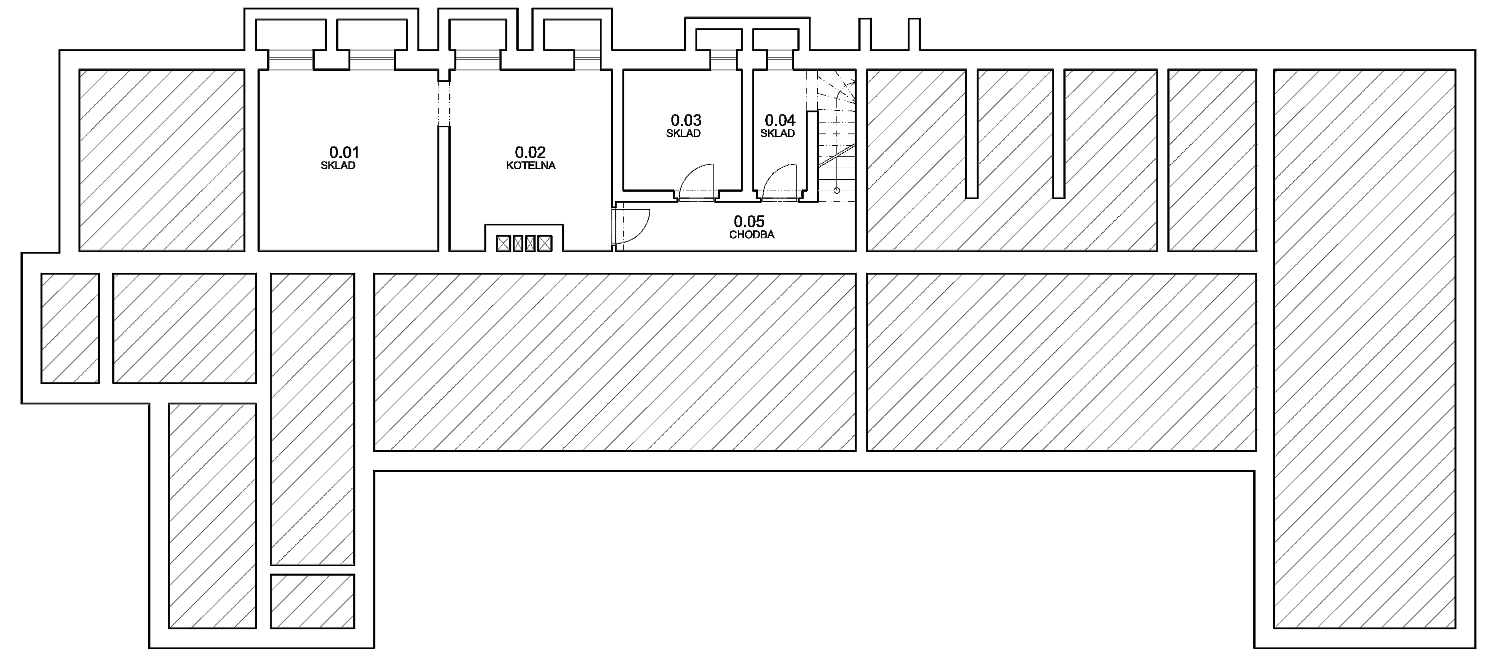
PŮDORYS 1.PP
